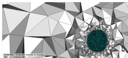
Fig.1b – Particolare mesh tetraedri in prossimità dell'oggetto
